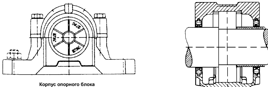
Корпус опорного блока
